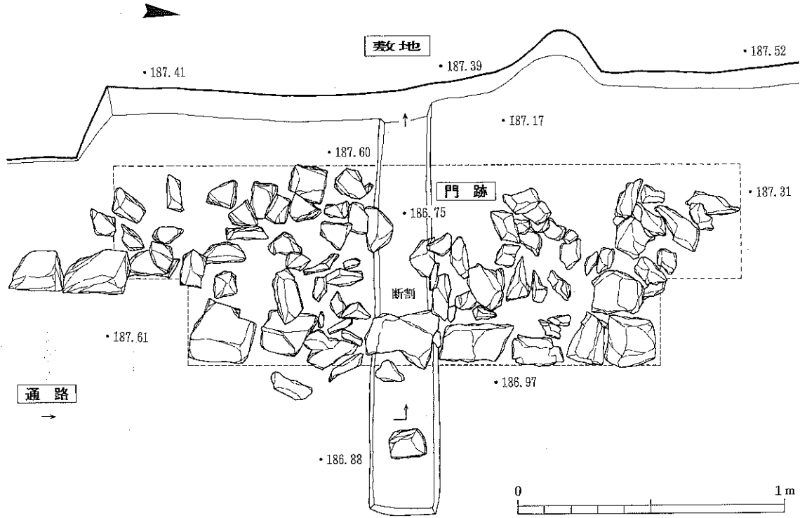
第 22 図 門跡平面実測図
