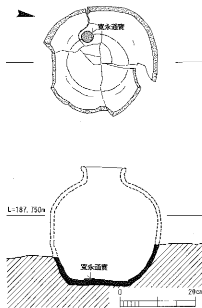
第 20 図 S X02 実測図
