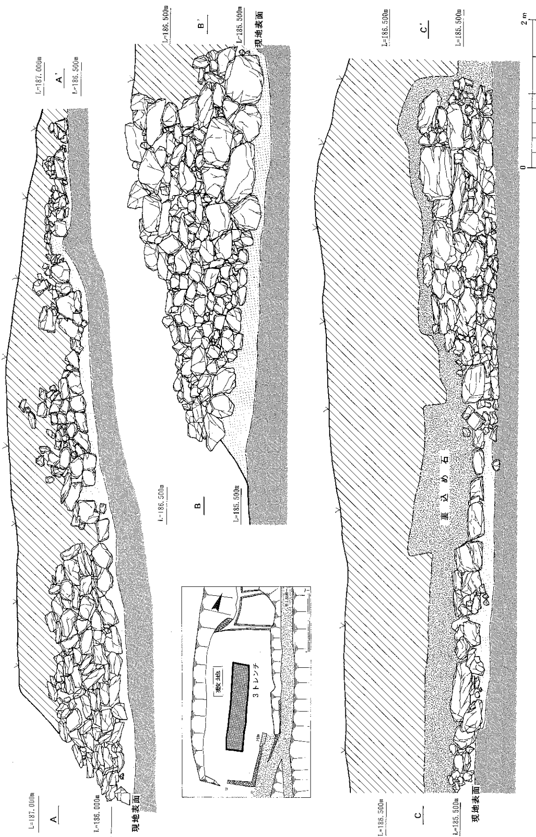
第24図 東側石垣（口道に接する）立面図
