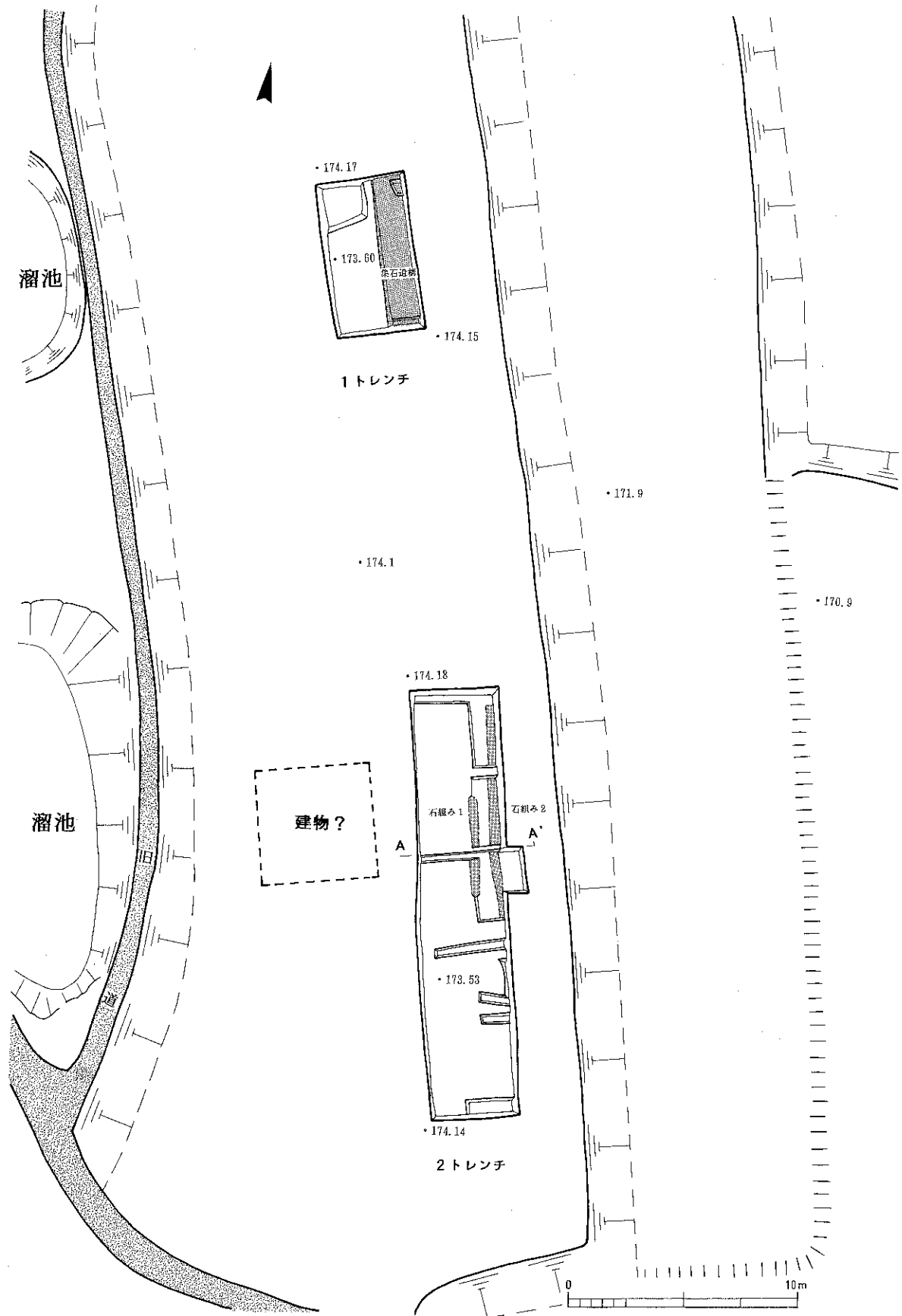
第31図 1・2トレンチ平面実測図
