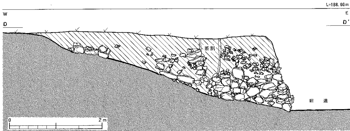
第29図 南側石垣立面図
