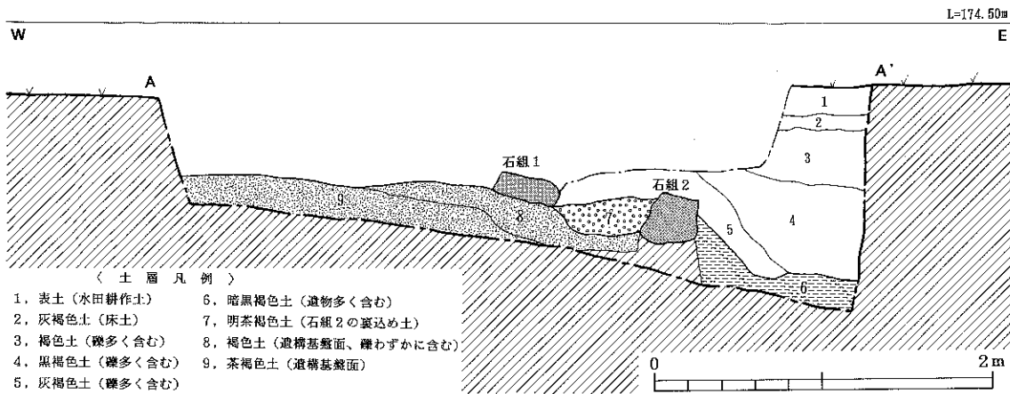
第34図 2トレンチ石組1・2の土層関係図
