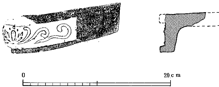
第24図 軒平瓦実測図
