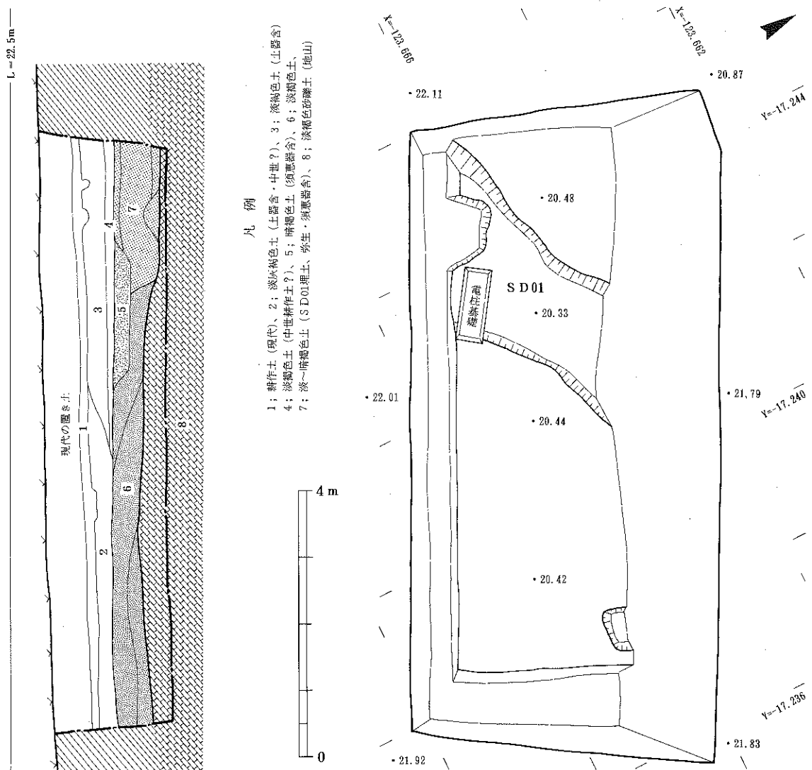
第23図 第2トレンチ実測図
