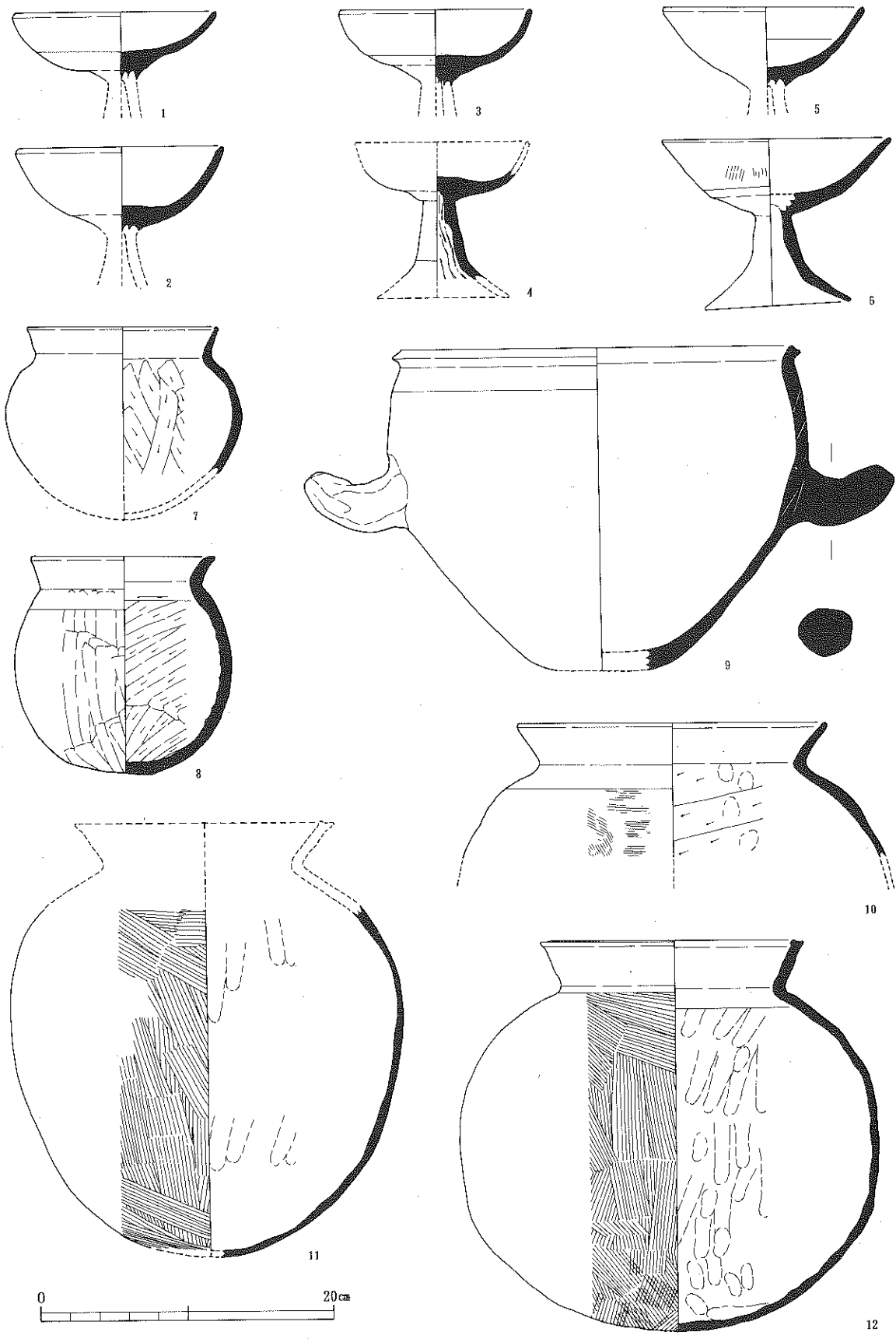
第24图 土城SK10出土土器实测图
