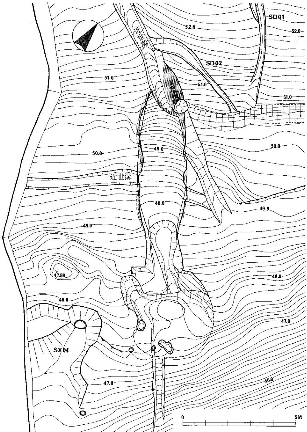
図版第五 遺構実測図3 (2号窯平面図)
