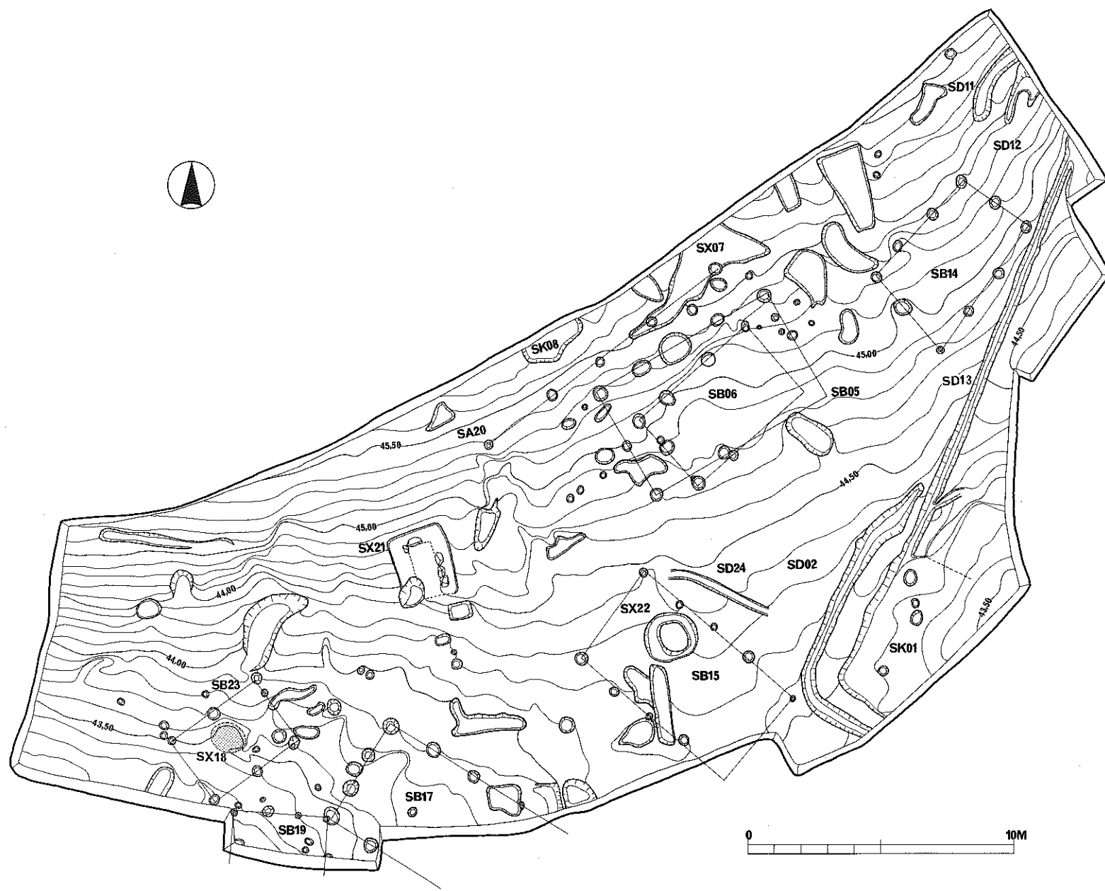
図版第九 遺構実測図7 (工房跡) (第3トレンチ平面図)
