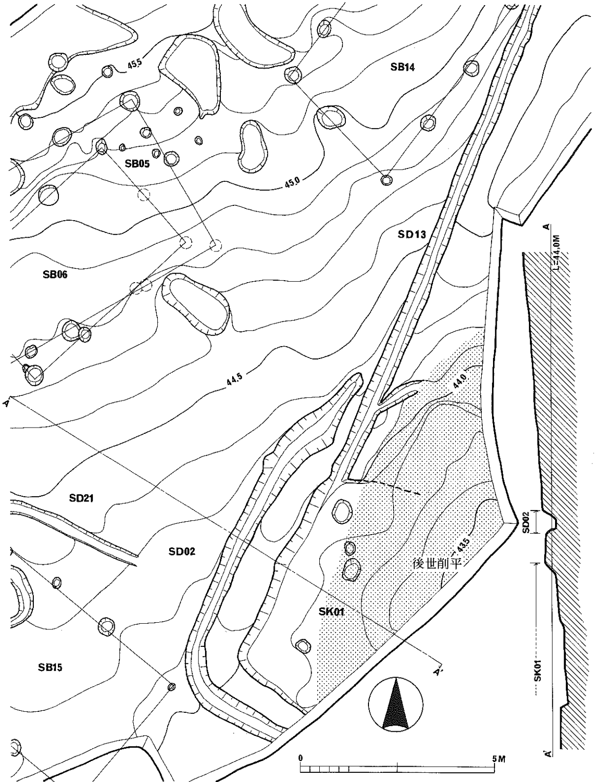
図版第一一 遺構実測図9〔工房跡〕(第3トレンチSK01・SD02・SD13実測図)
